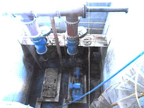
Foto 38 – Bombas para recalque Fonte: PROJEC.
