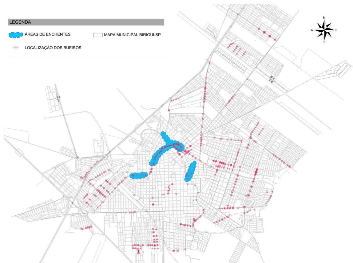
Figura 27 – Localização dos bueiros e das áreas de enchentes Fonte: PROJEC (2015)
